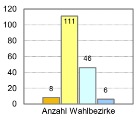
Häufigkeitsverteilung
