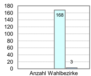
Häufigkeitsverteilung
