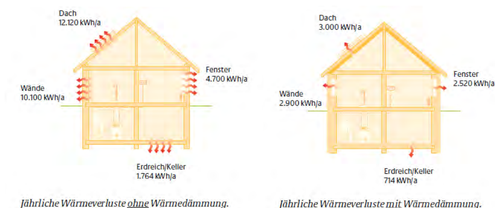
Abbildung 3.1: Durchschnittliche Wärmeverluste von Gebäuden [Quelle: DENA 2009]
